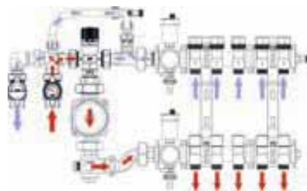
Рис. 5 – Распределение потоков
