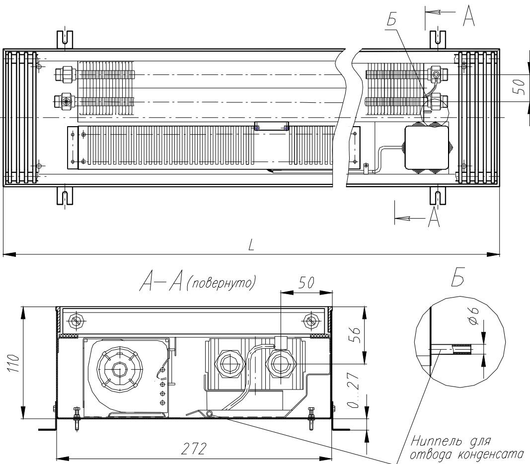
Рис. 1.4. Конвектор КВОК концевой с правосторонним подключением
