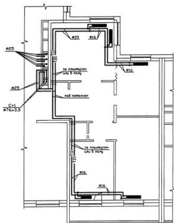
Рис. 2.1. Система отопления поквартирная двухтрубная горизонтальная
