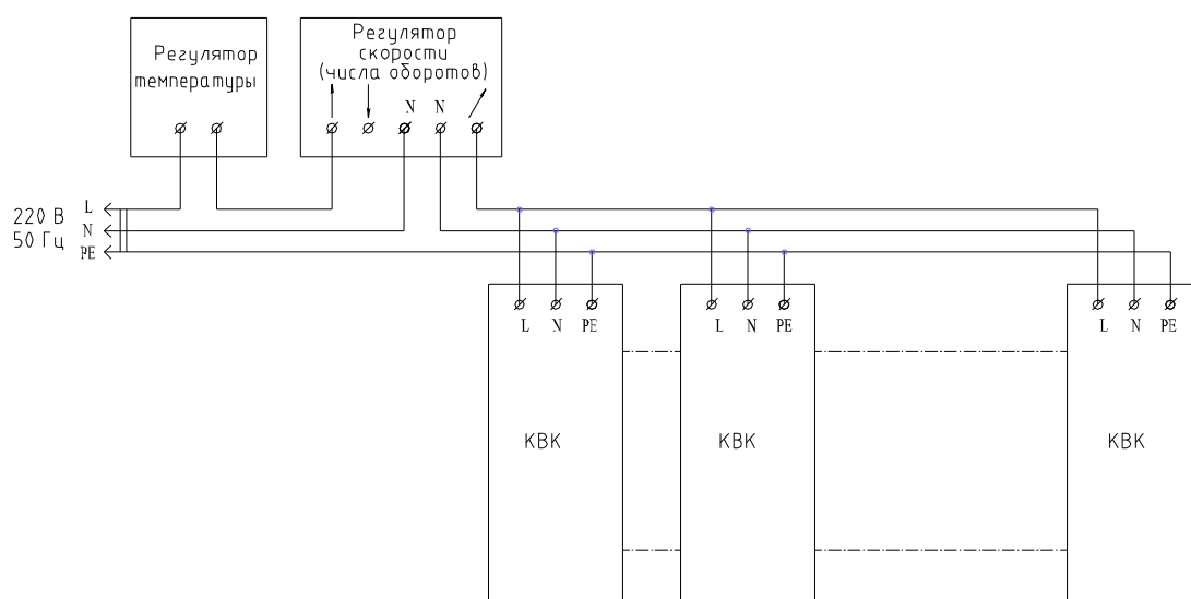
Рис.2.3 Схема подключения регулятора скорости и температуры.
